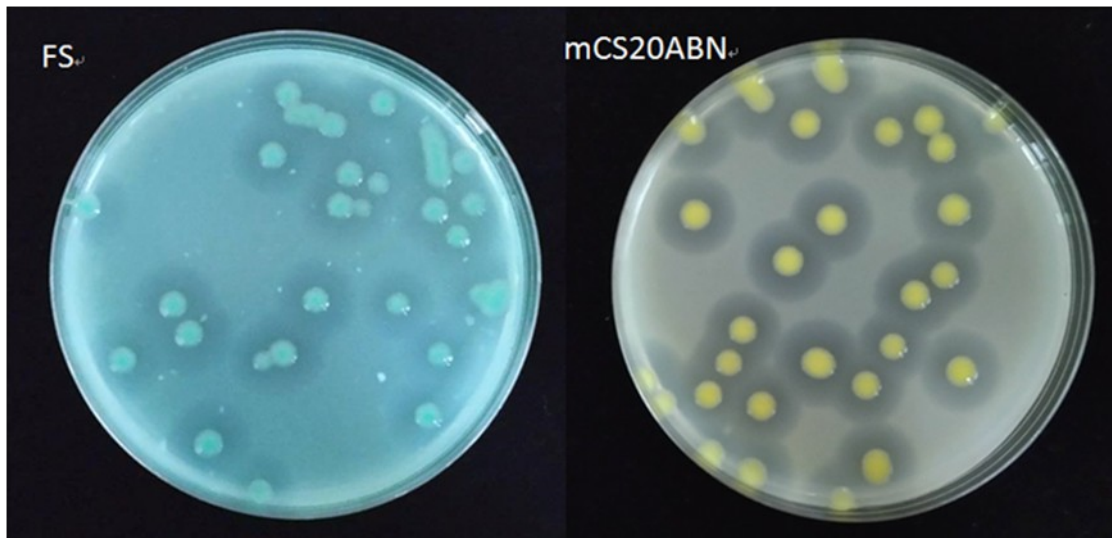
圖一、培養後 7 天， Xcc 及 Xcr 在 mFS 半選擇性培養基上呈淡綠色黏稠狀菌落，在 mCS20ABN 半選擇性培養基上呈淡黃色黏稠狀菌落，周圍皆可見有澱粉水解透化圈。
